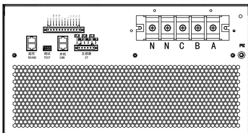
图 2-3 端口配置图
