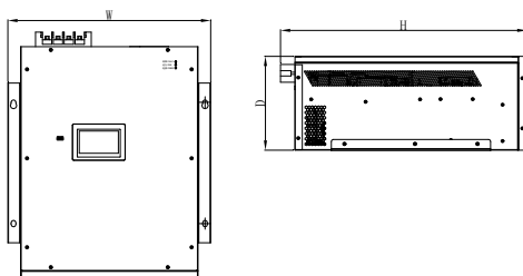
壁挂式 SVG 外形图
