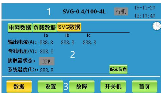
图 4-2 LCD 触摸屏内部界面示意图
