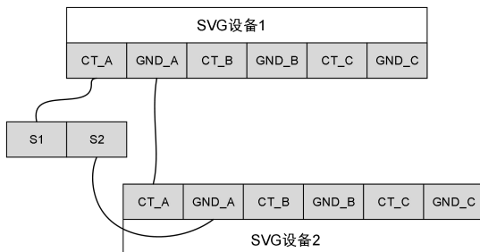
图 3-4 并机时的 CT 串联接法
