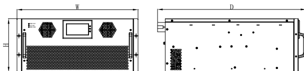
机架式 SVG 外形图
